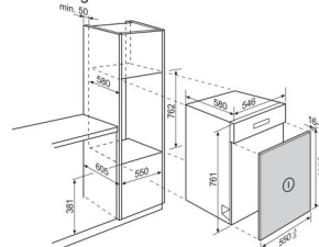
GA55LI/GLI/SLI - eingebaut in Hochschrank
