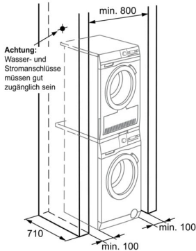
Belüftungsbeispiel für Wasch-Trockensäule, Nischeneinbau
