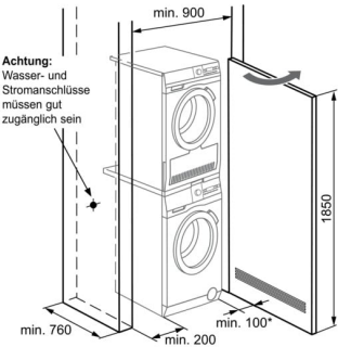
Belüftungsbeispiel für Wasch-Trockensäule, Nischeneinbau mit einfahrbarer Tür Tür muss bei Betrieb geöffnet sein (Belüftung in Türe integriert)
