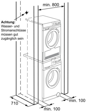
Belüftungsbeispiel für Wasch-Trockensäule, Nischeneinbau
