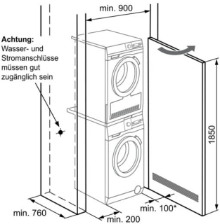
Belüftungsbeispiel für Wasch-Trockensäule, Nischeneinbau mit einfahrbarer Tür Tür muss bei Betrieb geöffnet sein (Belüftung in Tür integriert)
