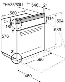
Einbaubackofen/Einbauherd + Höhenadapter EB6.../EH6... + HA35/60U
